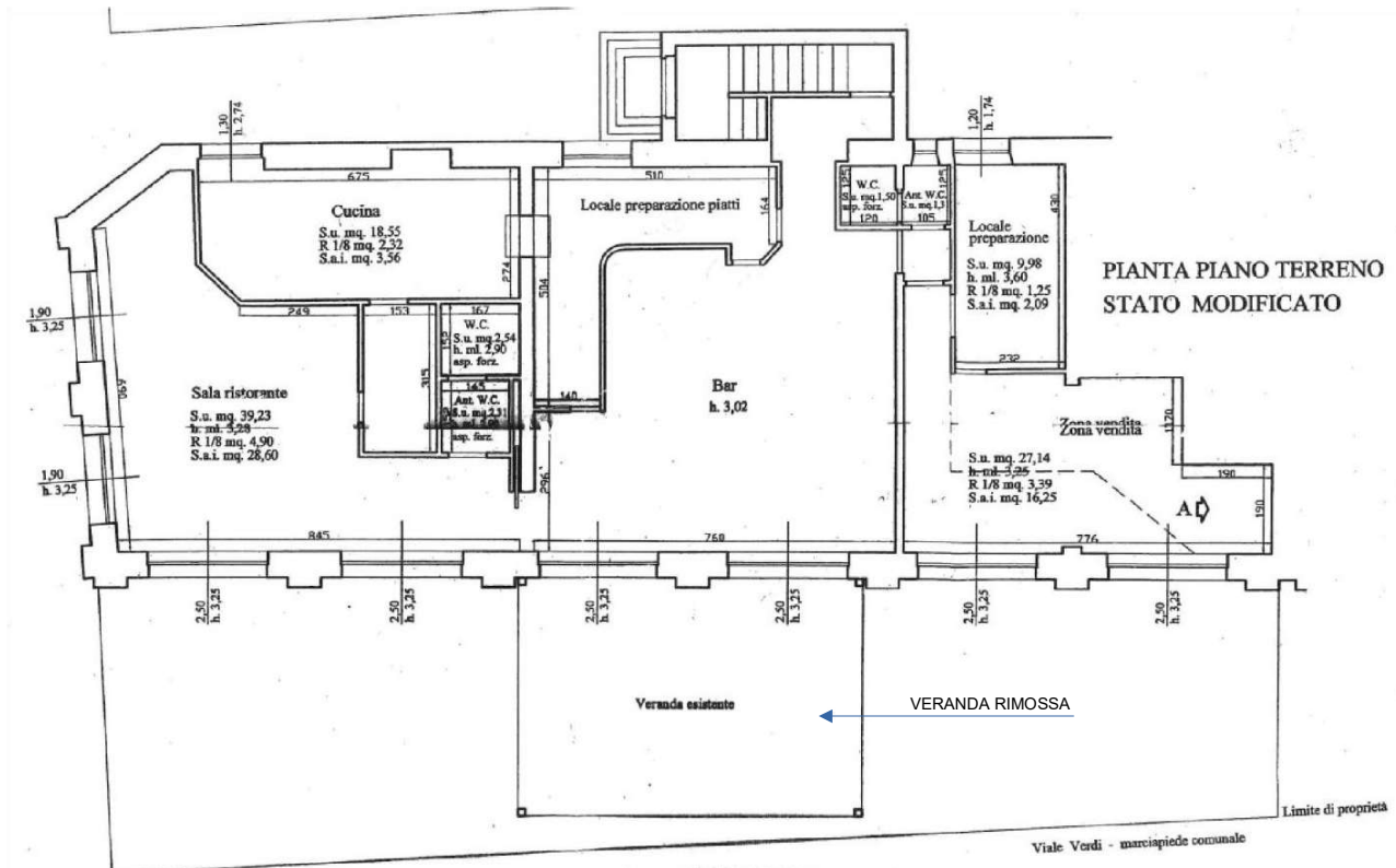
PIANTA PIANO TERRA Estratto Pratica Edilizia n. 2013/0021L
